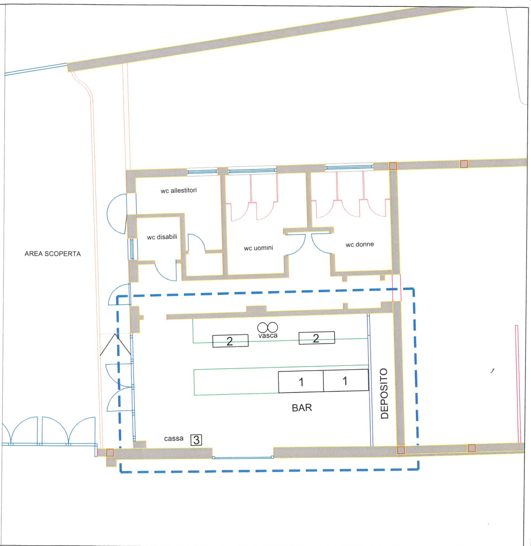
PLANIMETRIA PUNTO BAR "MIMOSA" - PADIGLIONE ESPOSITIVO 1 - (g)
